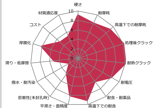
TAF TR
