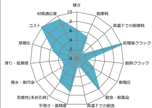
硫酸アルマイト
